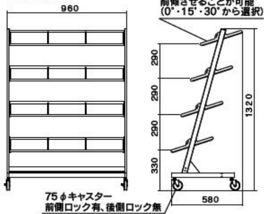
バスケットラック 4段 本体部寸法図
